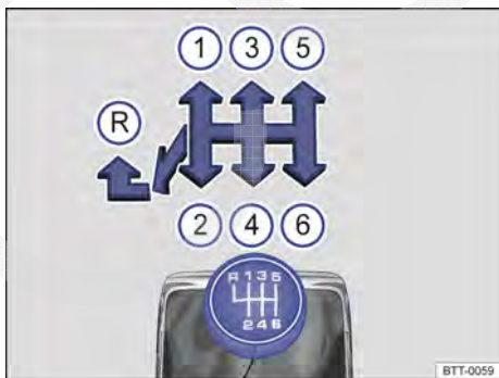
Fig. 112 Esquema de troca de marchas da transmissão manual de 6 velocidades.
