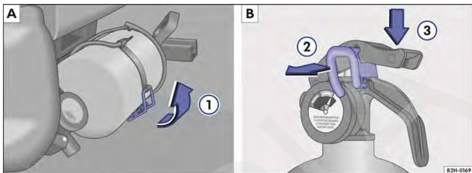
Fig. 166 A: no banco do passageiro dianteiro: localização do extintor de incêndio. B: sequência de operação.
