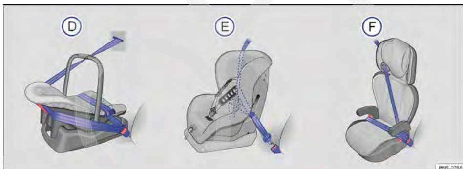
Fig. 71 As figuras (D), (E) e (F) mostram como o sistema de retenção para crianças é fixado somente com o cinto de segurança do veículo.
