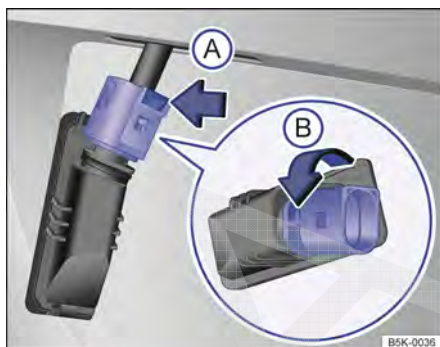
Fig. 200 Lanterna da placa licença: desinstalar o suporte da lâmpada.
