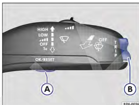
Fig. 12 Veículos sem volante multifunções: botão (A) na alavanca dos limpadores do para-brisa para confirmar itens de menu e chave (B) para trocar menus.
