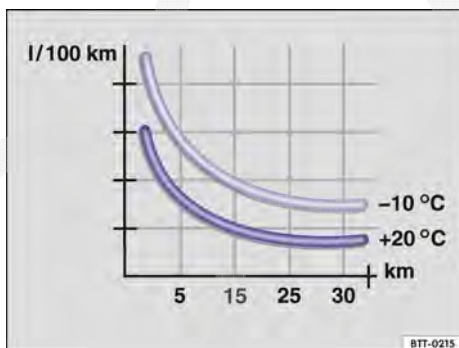
Fig. 119 Consumo de combustível em l/100 km em 2 temperaturas ambiente diferentes.
