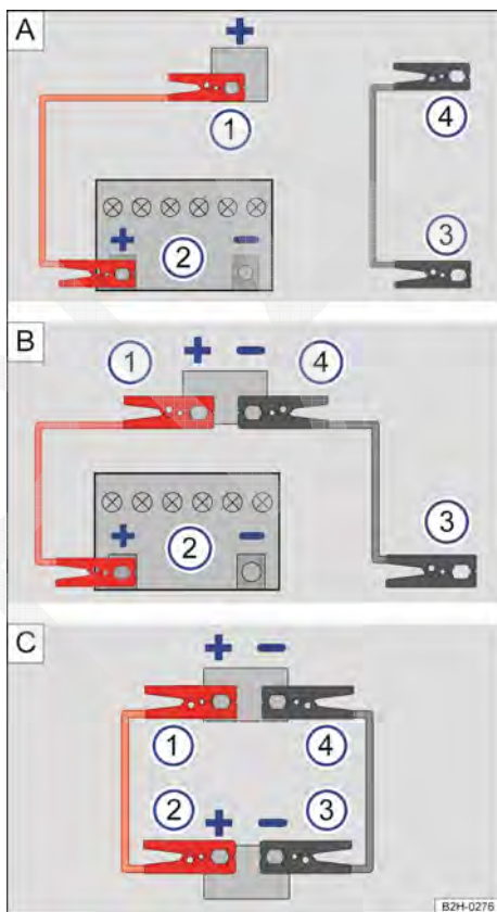
Fig. 207 No compartimento do motor: conexões para o cabo de auxílio à partida (representação esquemática).
