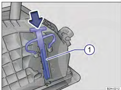
Fig. 172 Embaixo da cobertura do quadro da alavanca cobertura: destravamento de emergência do bloqueio da alavanca seletora.
