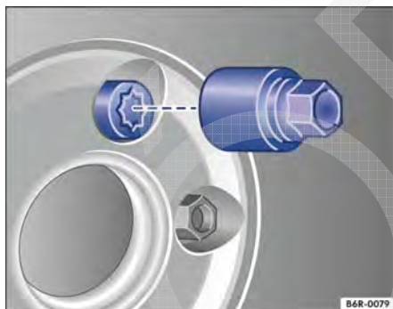
Fig. 181 Troca de roda: Parafusos de roda antifurto e adaptador.
