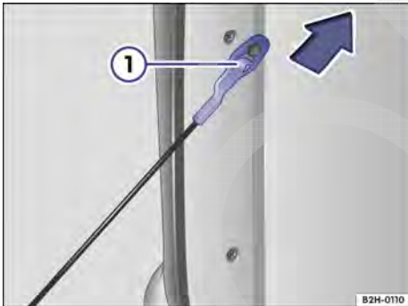
Fig. 24 Desprender os cabos de sustentação da tampa do compartimento de carga.
