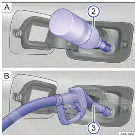
Fig. 138 Representação esquemática: abastecimento com AdBlue.
