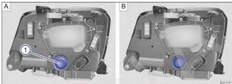
Fig. 194 No compartimento do motor: cobertura no farol de xenônio dianteiro direito: Ⓜ️ indicador de direção.
