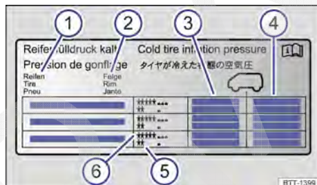
Fig. 158 Indicações na etiqueta com as pressões dos pneus.
