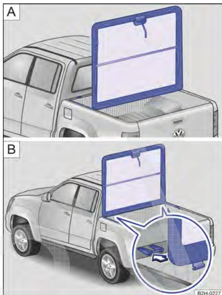
Fig. 26 Cobertura do compartimento de carga A : remover a cobertura do compartimento de carga para trás e B : posicionar a cobertura do compartimento de carga sobre os eixos dos suportes.
