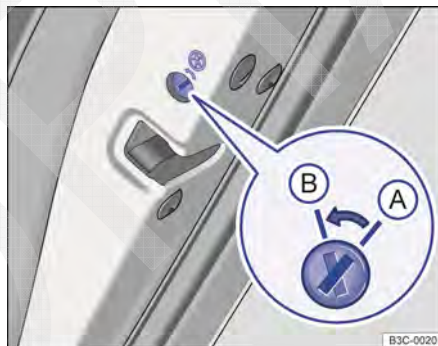
Fig. 22 Na porta traseira direita: trava de segurança para crianças (A) desativada, (B) ativada.
