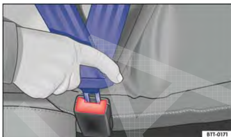
Fig. 55 Introduzir a lingueta do cinto de segurança no fecho do cinto de segurança.
