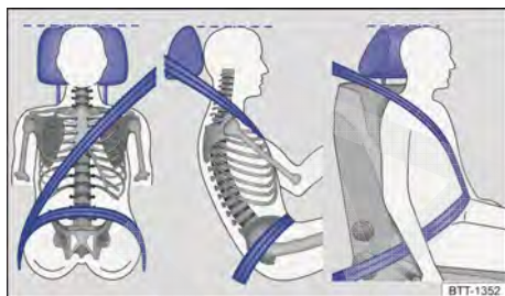
Fig. 61 Posição correta do cadarço do cinto de segurança e ajuste correto do apoio para cabeça.
