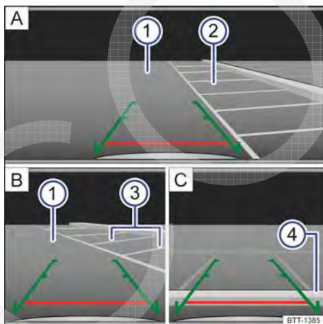
Fig. 124 Exibição do display do sistema Infotainment: entrar na vaga de estacionamento com a câmera de marcha a ré. A , Procurar vaga de estacionamento, B , dar o comando para a vaga de estacionamento selecionada, C , manobrar.
