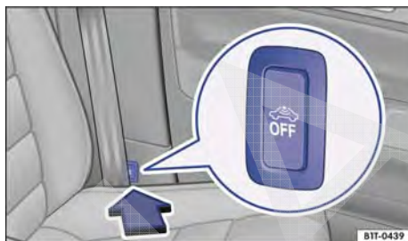
Fig. 20 Ao lado do banco do condutor: botão para desligar o monitoramento do interior do veículo e o alarme antirrebocagem.
