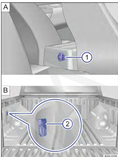
Fig. 107 Tomada 12 V: no console central traseiro ③ e no compartimento de carga ④.
