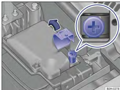
Fig. 205 No compartimento do motor: polo positivo do ponto de auxílio à partida.
