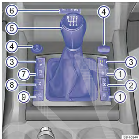
Fig. 9 Vista geral da parte frontal do console central (veículos com direção à direita).
