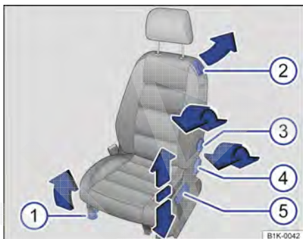
Fig. 35 Comandos do banco dianteiro esquerdo.
