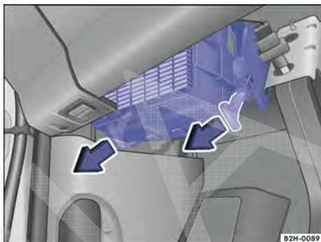
Fig. 189 Caixa de fusíveis abaixo do painel de instrumentos (veículos com direção à esquerda).
