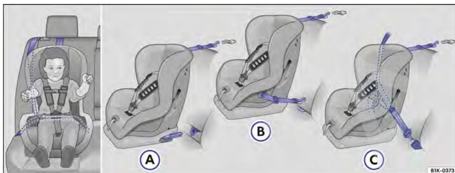
Fig. 70 No banco traseiro: as figuras (A) e (B) mostram como o sistema de retenção para crianças é fixado nos olhais de suporte inferiores e com o cinto de fixação superior. A figura (C) mostra como o sistema de retenção para crianças é fixado com o cinto de segurança do veículo e com o cinto de fixação superior.
