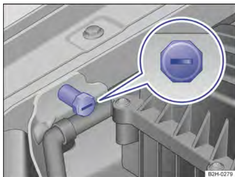
Fig. 206 No compartimento do motor: ponto negativo do ponto de auxílio à partida.
