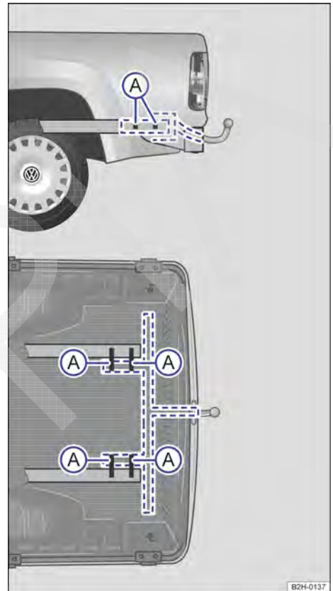
Fig. 95 Veículos sem para-choque: pontos de fixação para instalação posterior de um dispositivo de reboque.
