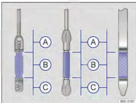
Fig. 147 Vareta de medição do óleo do motor com marcas de nível de óleo do motor.
