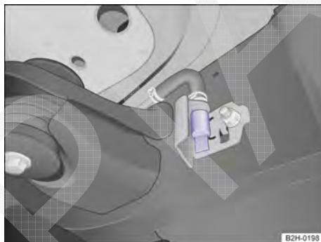
Fig. 136 Parte inferior do veículo na longarina do lado esquerdo do veículo: bujão de drenagem.
