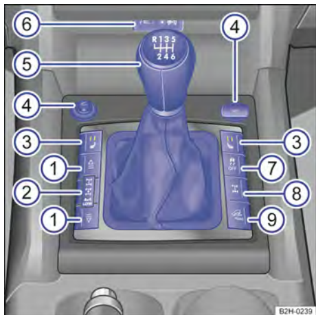
Fig. 8 Vista geral da parte frontal do console central (veículos com direção à esquerda).
