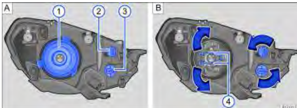
Fig. 148 No compartimento do motor: vista traseira do farol dianteiro esquerdo com cobertura de borracha: ① farol baixo e farol alto, ② luz de posição, ③ indicadores de direção e trava de proteção ④.
