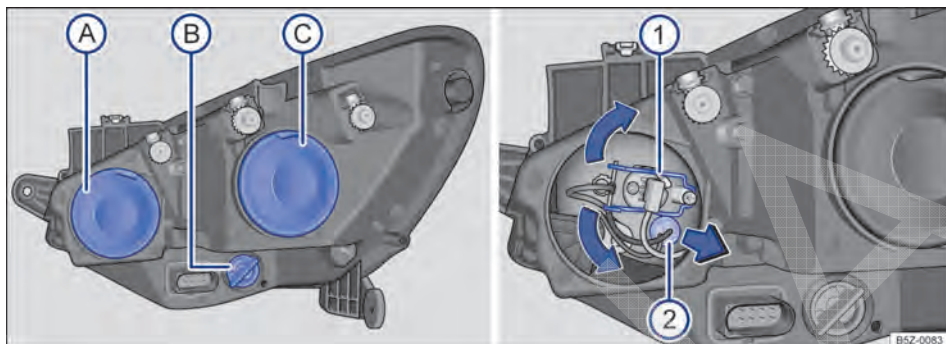
Fig. 173 No compartimento do motor: vista traseira do farol dianteiro direito com cobertura de borracha (esquerda): A farol alto e luz de posição, B indicadores de direção e C farol baixo. Vista traseira do farol dianteiro direito sem cobertura de borracha (direita): 1 farol alto, 2 luz de posição.
