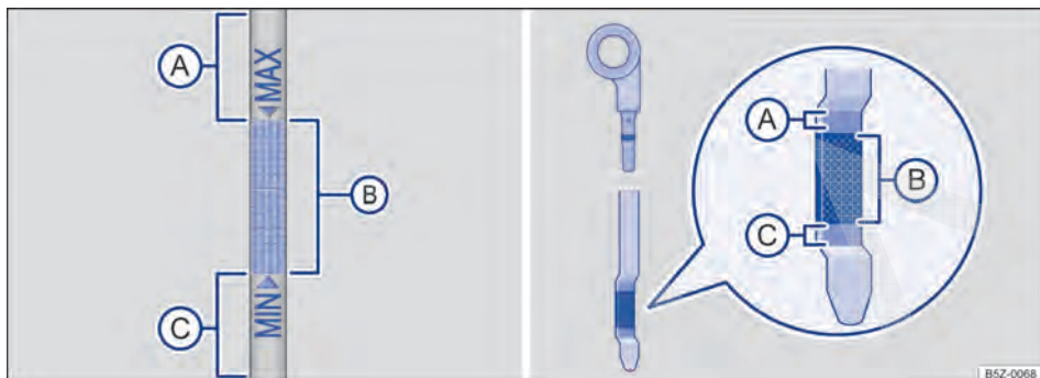
Fig. 130 Vareta de medição do óleo com marcas de nível do óleo do motor.
