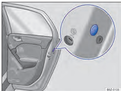
Fig. 159 Na porta traseira: travamento de emergência, coberto por uma vedação de borracha.
