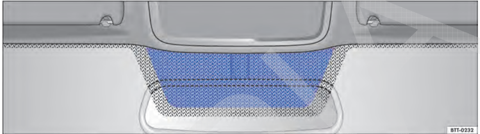
Fig. 61 Para-brisa com infravermelho e revestimento metálico com janela de comunicação (superfície azul).
