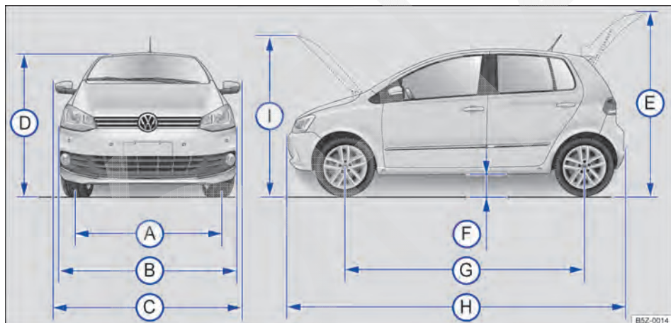
Fig. 194 Dimensões.
