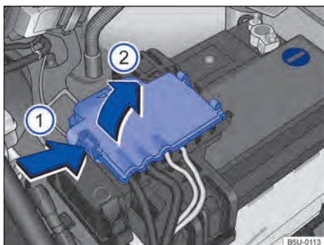
Fig. 165 Compartimento do motor: acesso ao terminal positivo da bateria.
