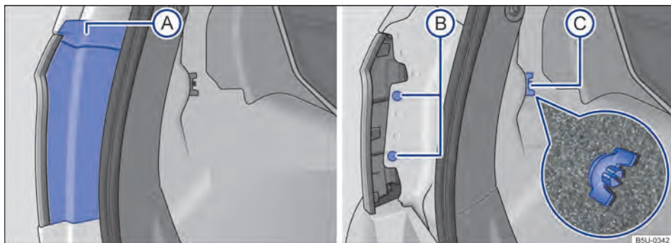
Fig. 155 No compartimento de bagagem: A desinstalar cobertura, B retirar os dois parafusos de fixação e C retirar o parafuso borboleta (lupa).
