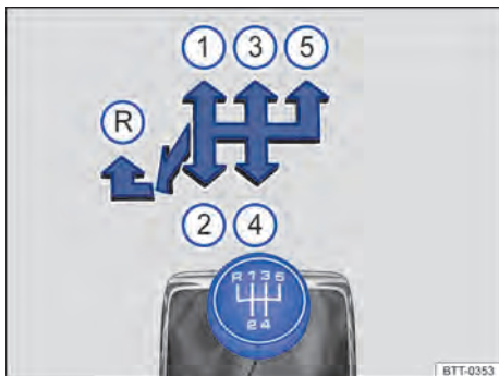
Fig. 81 Esquema de troca de marchas da transmissão manual de 5 marchas.
