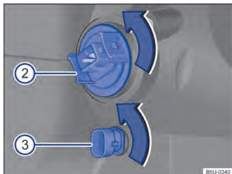
Fig. 151 No compartimento do motor: vista traseira do farol dianteiro 2 indicadores de direção e 3 luz de posição.
