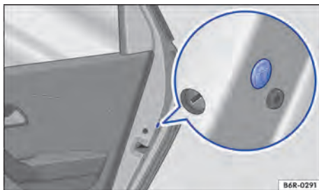
Fig. 48 Na porta traseira: travamento de emergência, coberto por uma vedação de borracha.
