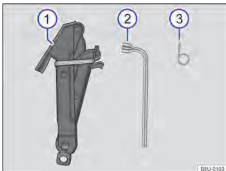
Fig. 145 Componentes das ferramentas de bordo.
