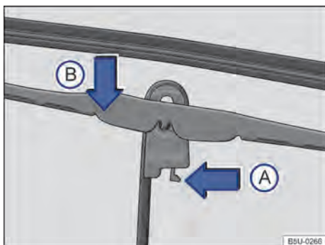
Fig. 146 Substituir as palhetas dos limpadores do para-brisa.
