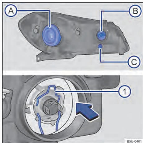
Fig. 150 No compartimento do motor: vista traseira do farol dianteiro com cobertura de borracha (lado esquerdo da ilustração) - A farol baixo / alto, B indicadores de direção e C luz de posição. Vista traseira do farol dianteiro sem a cobertura de borracha (lado direito da ilustração): 1 mola de travamento da lâmpada incandescente do farol baixo / alto.
