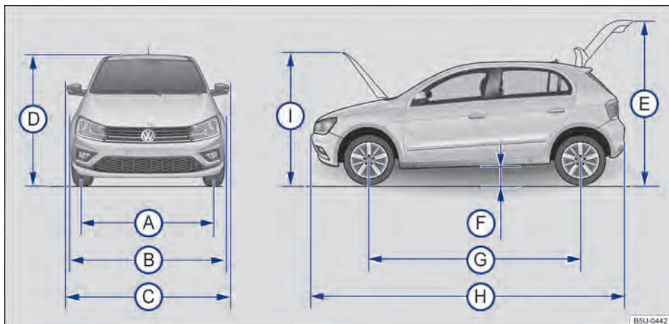
Fig. 193 Dimensões.
