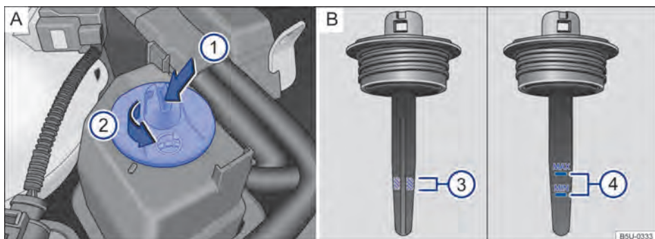
Fig. 86 No compartimento do motor (variante 1): A ) Reservatório do fluido da direção hidráulica. B ) Marcações para controle do nível do fluido da direção hidráulica.
