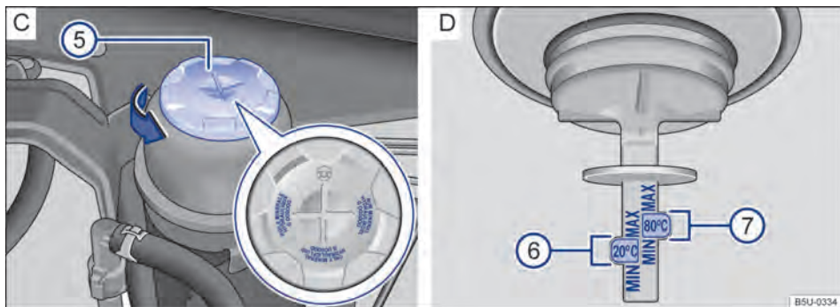
Fig. 87 No compartimento do motor (variante 2): C ) Reservatório do fluido da direção hidráulica. D ) Marcações para controle do nível do fluido da direção hidráulica.
