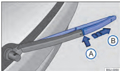
Fig. 147 Substituir a palheta do limpador do vidro traseiro.
