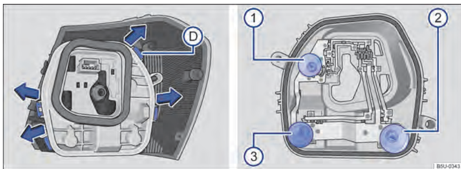
Fig. 156 Lanterna traseira: D desinstalar o suporte das lâmpadas e 1 , 2 e 3 desinstalar as lâmpadas.
