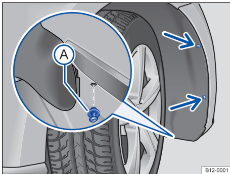
Fig. 111 Na caixa da roda dianteira direita: remover os parafusos de fixação (setas) e remover o rebite de expansão (A).
