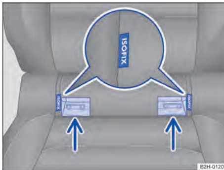
Fig. 8 No banco do veículo: variantes de identificação dos pontos de ancoragem inferiores para cadeiras de criança.
