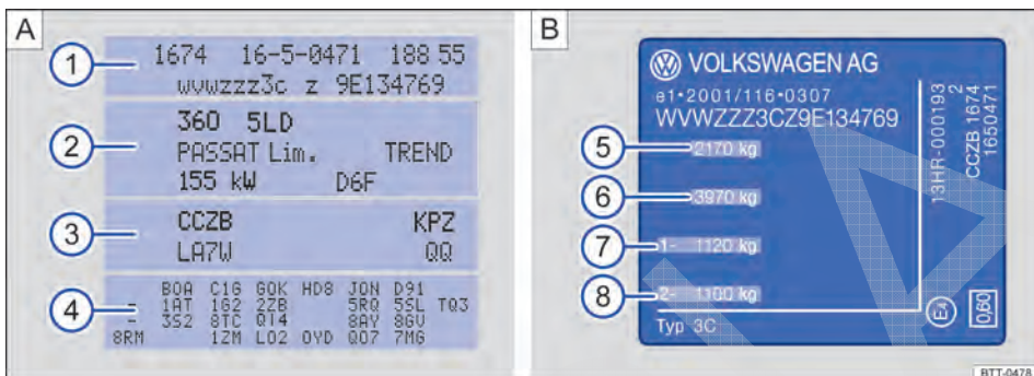
Fig. 1 (A) Etiqueta de dados do veículo: o exemplo na figura mostra as letras do código de um motor CCZB (3). (B) Etiqueta de características do veículo.
