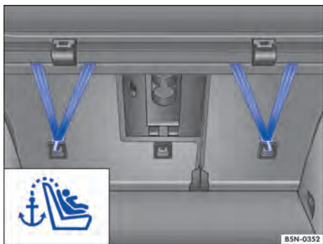
Fig. 9 Cintos de fixação superiores encaixados no compartimento de bagagem.
