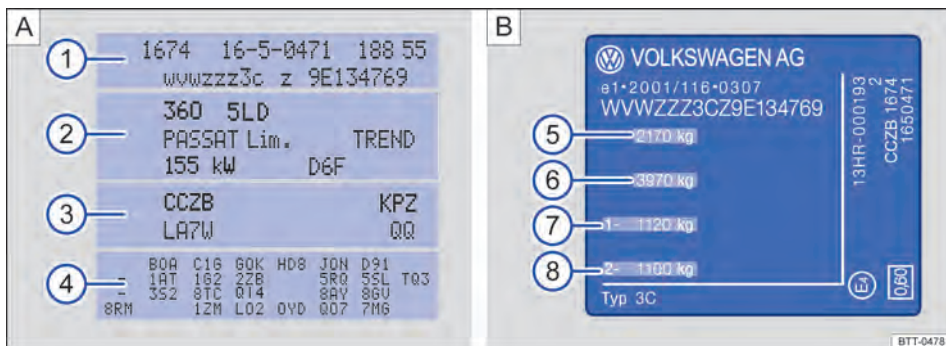
Fig. 2 (A) Etiqueta de dados do veículo: o exemplo na figura mostra as letras do código de um motor CCZB (3). (B) Etiqueta de características do veículo.
