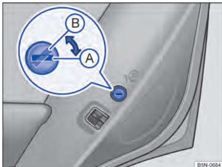
Fig. 11 Na porta traseira direita: trava de segurança para crianças (A) desativada, (B) ativada.
