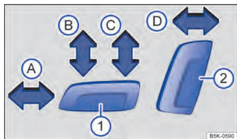
Fig. 72 Interruptor no banco dianteiro esquerdo: ajustar o banco dianteiro esquerdo na longitudinal, o assento do banco em altura e inclinação, bem como o encosto do banco dianteiro.
