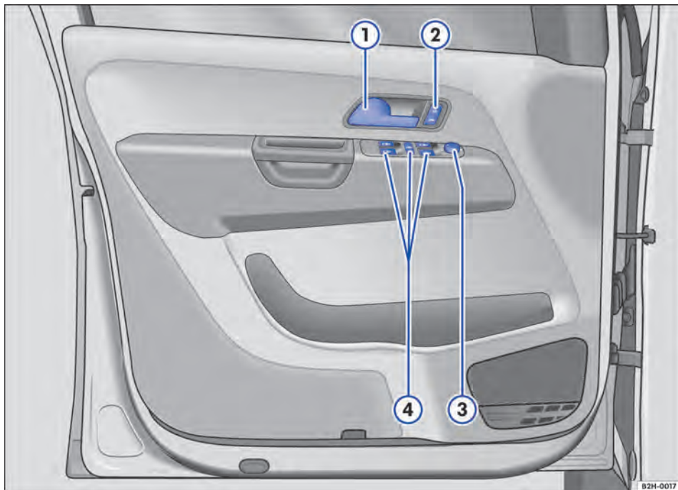
Fig. 6 Vista geral dos elementos de comando na porta do condutor (veículos com direção à esquerda).
