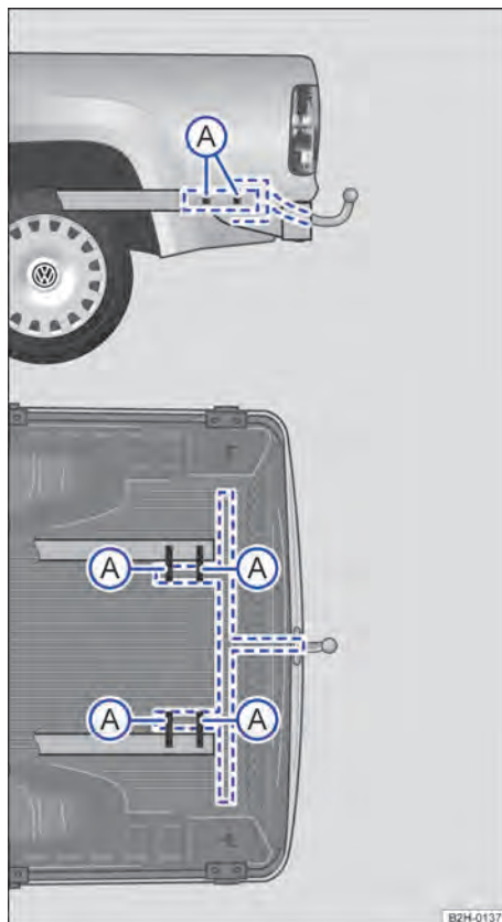
Fig. 149 Veículos sem para-choque: pontos de fixação para instalação posterior de um dispositivo de reboque.
