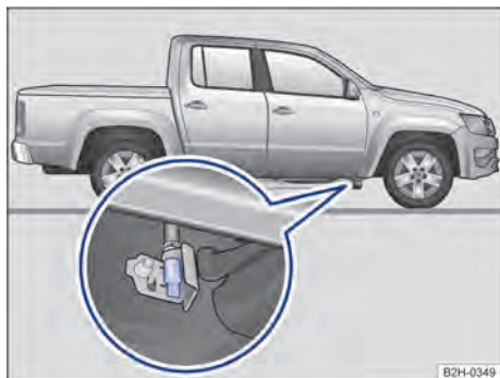
Fig. 152 Na parte inferior do veículo, na longarina: bocal de drenagem do filtro de óleo diesel (dependendo da versão).
