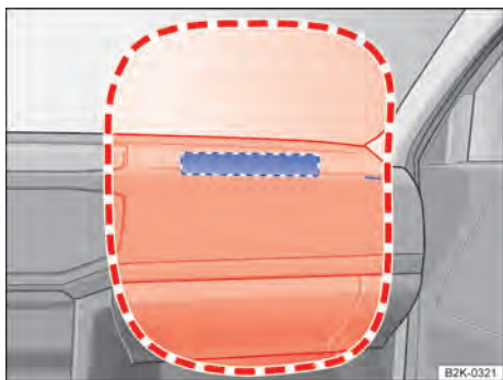
Fig. 48 Local de instalação e área de expansão do airbag dianteiro do passageiro dianteiro.
