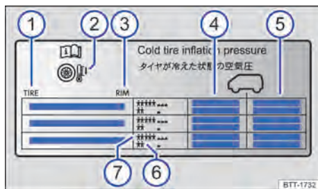
Fig. 195 Indicações na etiqueta de pressão dos pneus.
