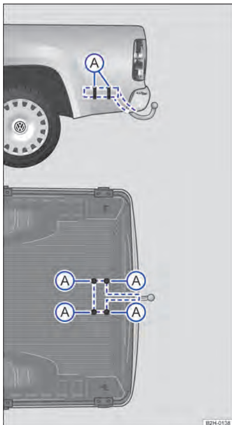
Fig. 150 Veículos com para-choque: pontos de fixação para a instalação posterior de um dispositivo de reboque.
