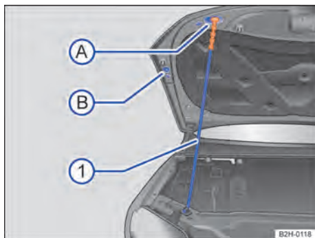
Fig. 180 Fixar a tampa do compartimento do motor com a haste de sustentação (representação esquemática).
