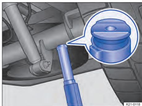
Fig. 216 Posicionar o macaco sob o eixo traseiro.
