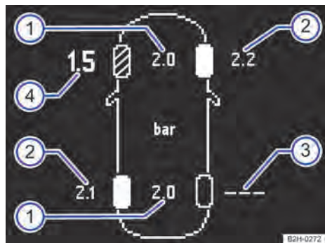
Fig. 192 Representação esquemática do indicador do display do instrumento combinado: pressões dos pneus atuais.
