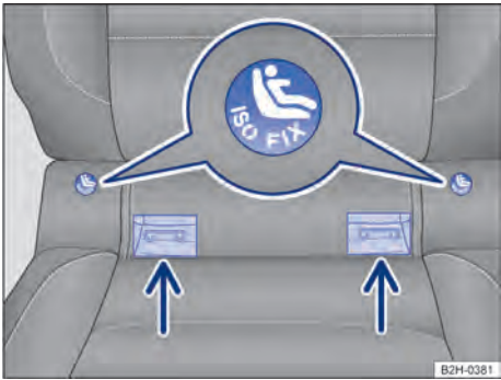
Fig. 55 No banco do veículo: identificação dos pontos de ancoragem inferiores para cadeiras de criança.
