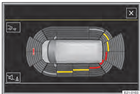
Fig. 119 No sistema Infotainment: detecção de obstáculos do auxílio ao estacionamento (representação esquemática).
