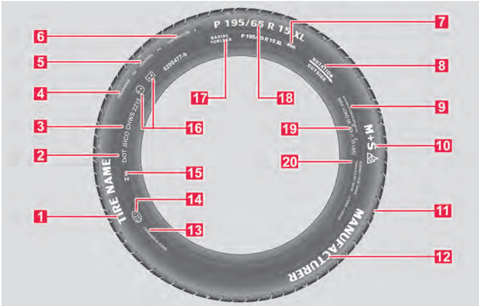
Fig. 198 Inscrição internacional dos pneus.
