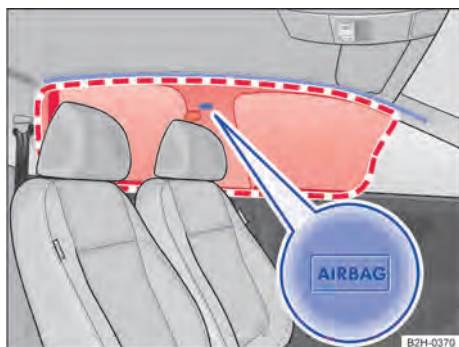
Fig. 52 No lado esquerdo do veículo: local de instalação e área de expansão do airbag para cabeça.
