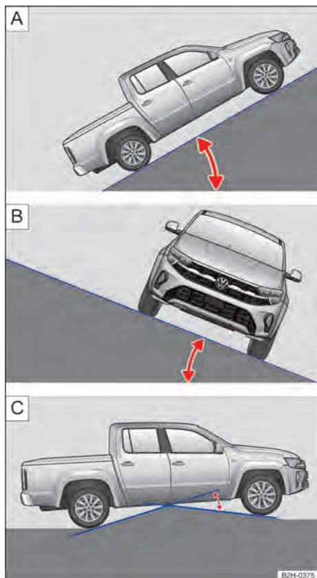
Fig. 112 Representação da rampa máxima [A], ângulo de inclinação [B] e ângulo de rampa [C].
