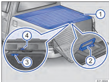
Fig. 67 Capota marítima do compartimento de carga: vista geral
