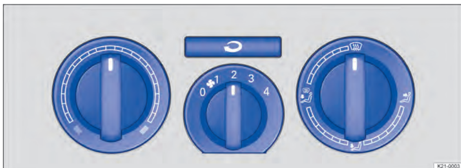
Fig. 99 No painel de instrumentos: elementos de comando do sistema de ventilação e aquecimento.
