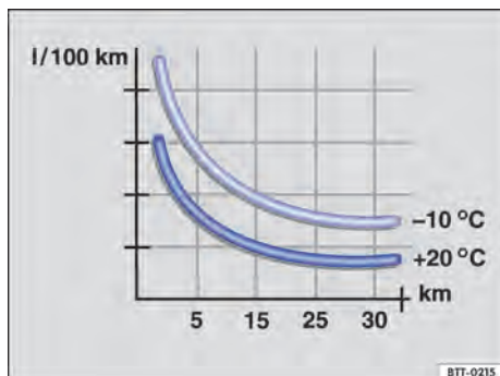
Fig. 103 Consumo de combustível em l/100 km em duas temperaturas-ambientes diferentes.
