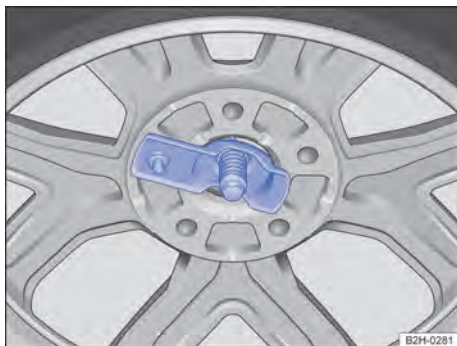
Fig. 207 Roda sobressalente ou de emergência: colocação correta do suporte do aro no orifício do aro.
