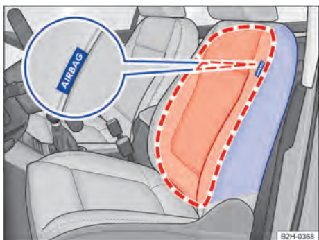
Fig. 51 Lateralmente no banco dianteiro: localização de instalação e área de expansão dos airbags laterais.
