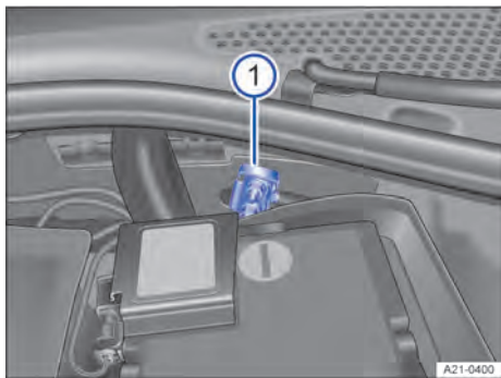
Fig. 171 No compartimento do motor: ponto de auxílio à partida (ponto de aterramento).
