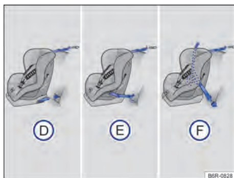
Fig. 54 No banco traseiro: as figuras D e E mostram o princípio da fixação do sistema de retenção para crianças nos olhais de retenção inferiores e com o cinto de fixação superior. A figura F mostra a fixação do sistema de retenção para crianças com o cinto de segurança do veículo e com o cinto de fixação superior.
