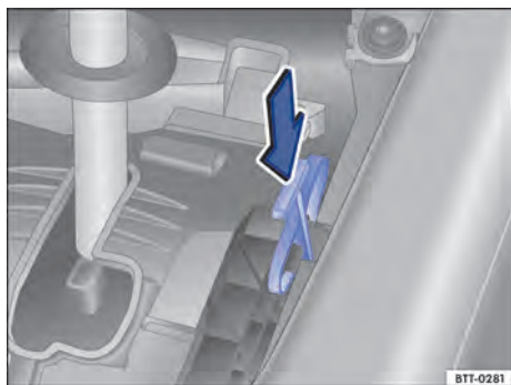
Fig. 109 destravar emergencialmente o bloqueio da alavanca seletora.
