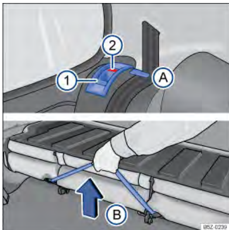
Fig. 63 Banco traseiro: botão de destravamento ①; posicionador para os cadarços dos cintos A; alça para destravamento do conjunto do assoalho B.
