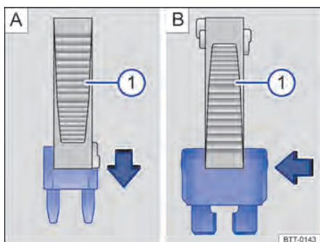
Fig. 166 Remover ou instalar um fusível com a garra da pinça de plástico ⓘ.
