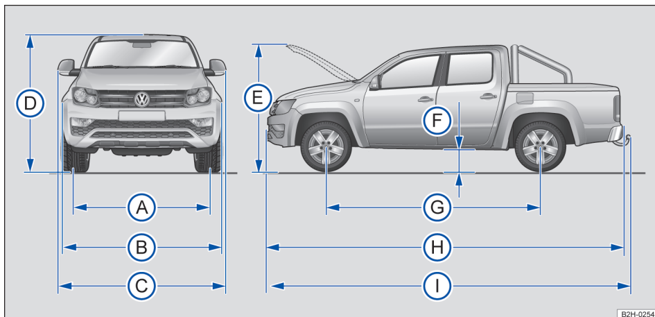
Fig. 13 Dimensões.
