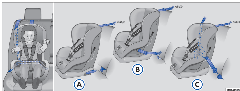
Fig. 2 No banco traseiro: as figuras A e B mostram o princípio da fixação do sistema de retenção para crianças nos olhais de retenção inferiores e com o cinto de fixação superior. A figura C mostra a fixação do sistema de retenção para crianças com o cinto de segurança do veículo e com o cinto de fixação superior.
