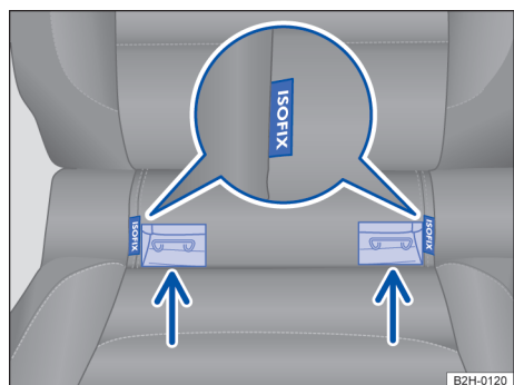
Fig. 6 No banco do veículo: variantes de identificação dos pontos de ancoragem inferiores para cadeiras de criança.
