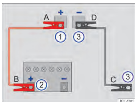
Fig. 211 Esquema para a conexão dos cabos auxiliares de partida no veículo que presta auxílio à partida (bateria do veículo 12 V no compartimento de bagagem).
