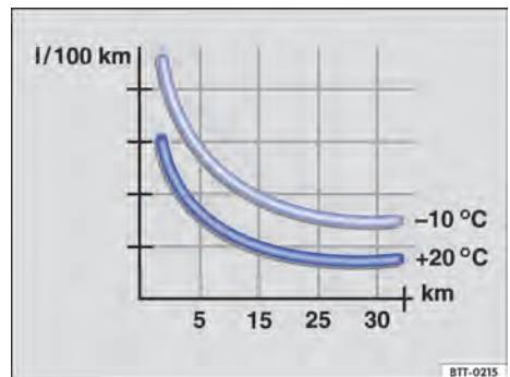
Fig. 116 Consumo de combustível em l/100 km em duas temperaturas ambiente diferentes.
