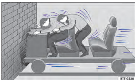
Fig. 32 Um veículo com os ocupantes do veículo sem cintos de segurança colide com o muro.
