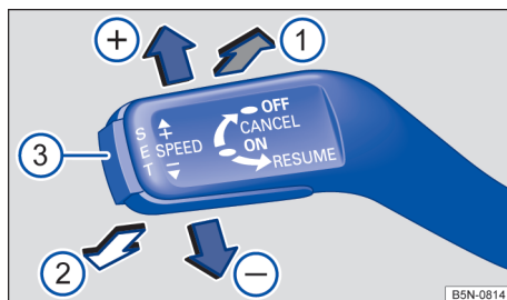
Fig. 137 À esquerda na coluna de direção: alavanca do GRA.
