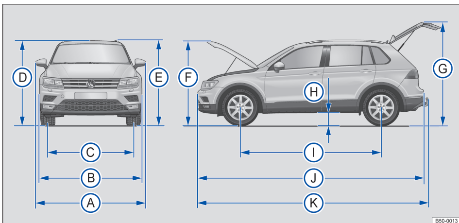
Fig. 252 Dimensões.
